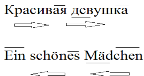
Рис. 3. Логика языка
