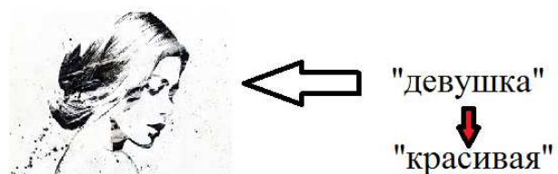
Рис. 2. Логика мысли
